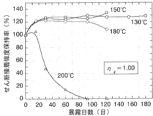
図11 熱劣化試験結果と、90℃~100℃3000日後の予測劣化係数 \eta_4
