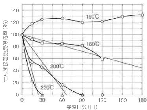
図8 熱劣化試験の一例
