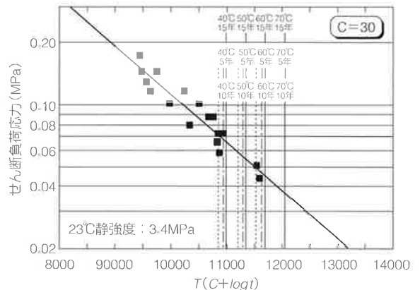
図12 Larson-Millerのマスターカーブ(直線)の一例
