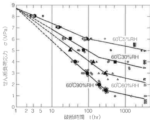
図7 60°Cにおける相対湿度とクリープ破断特性
