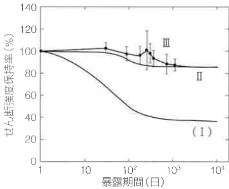
図10 乾燥による強度回復を考慮した屋外暴露劣化の推定結果(Ⅱ)と実測値(Ⅲ)の比較 [曲線(Ⅰ)はアレニウス法で求めた連続25℃多湿環境での劣化曲線]
