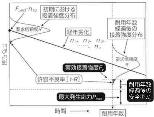
図13 接着強度の経年変化の概念図
