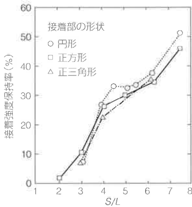
図5 S/Lと接着強度保持率の関係
